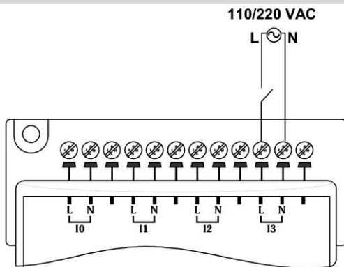
Câblage des entrées (groupe d'entrées du haut)
