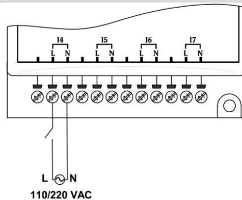
Câblage des entrées (groupe d'entrées du bas)
